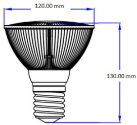
E39/41 Beam Angle 20°,38°,50°,90°,100°
