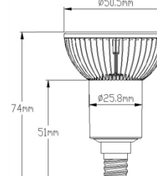
Design E12 (EURO)
